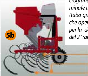
Figura 5b: vista laterale. Si noti nel particolare il posizionamento dei tubi di calata accoppiati.
