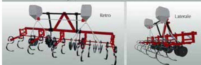
Figura 4: schema di montaggio di sarchiatore 4 file a telaio fisso, con installata attrezzatura per l'applicazione di ERCOLE ed il serbatoio di grande capacità per la distribuzione localizzata del fertilizzante in copertura. I microgranulatori vengono qui proposti con installazione anteriore rispetto al serbatoio del fertilizzante: il sistema degli assolcatori è configurato come schematizzato in Figura 3.
